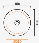
Sfera ø 45 cod. 145ASF00
