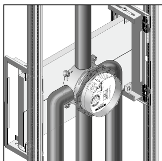
Montaža na sustave nosača
