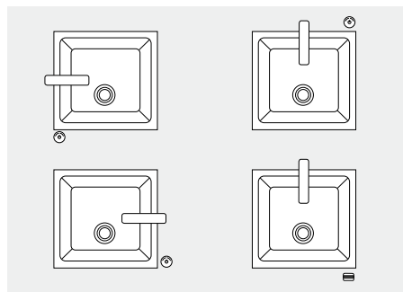
Primjeri za verzije ugradnje
