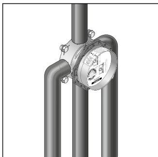
Instalacija izravno na zidu
