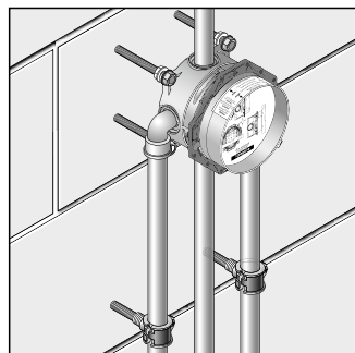
Instalacija ispred zida; ovdje s varijabilnim držačima razmaka pomoću dijana vijaka M10
