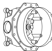
iBox® universal Osnovno tijelo iBox universal # 01800180 Set za produžetak 25 mm kod preduboke ugradnje: # 13595000 Set za produžetak 22 mm kod preplitke ugradnje: # 13596000 za rozete s promjerom 170 mm # 13597000 za rozete s promjerom 150 mm # 97407000 za rozete s promjerom 172 mm # 15597000 za PuraVida
