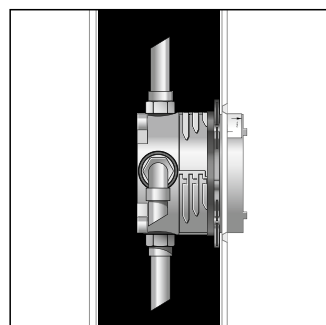
Montaža na gotove montažne ploče ili gotove elemente
